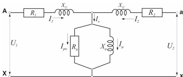
Sl. 5 – Ekvivalentna T šema transformatora
